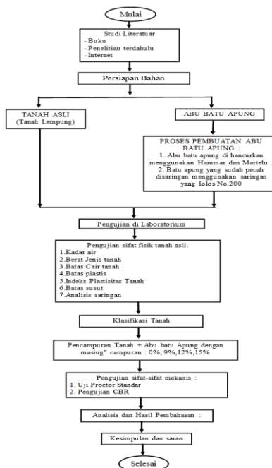
Gambar 1 Bagan Alir Penelitian Sumber : Data Excel pribadi 2024
