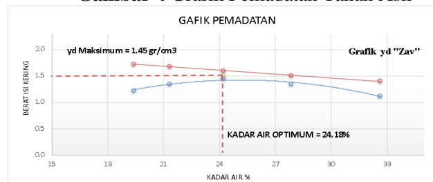
Gambar 4 Grafik Pemadatan Tanah Asli
