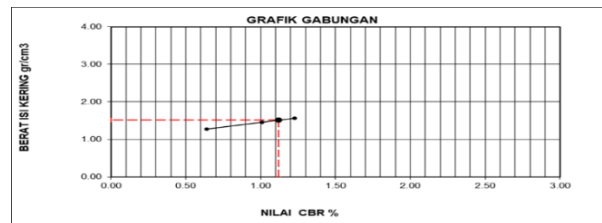
Gambar 2 Grafik CBR Tanah Asli
